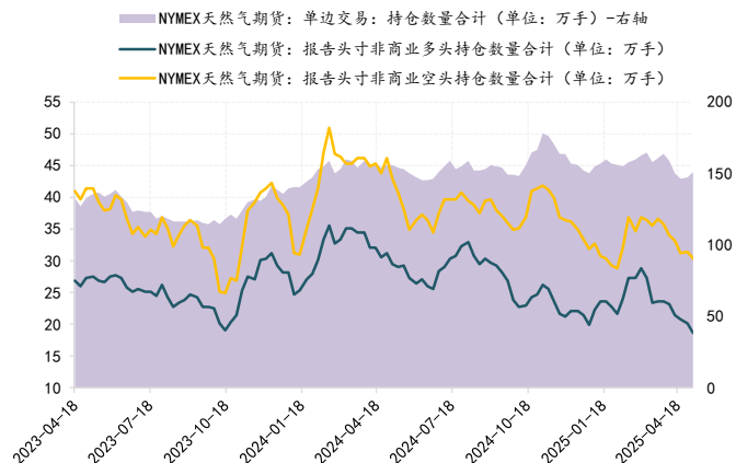
美气非商业多头/空头持仓数量情况
