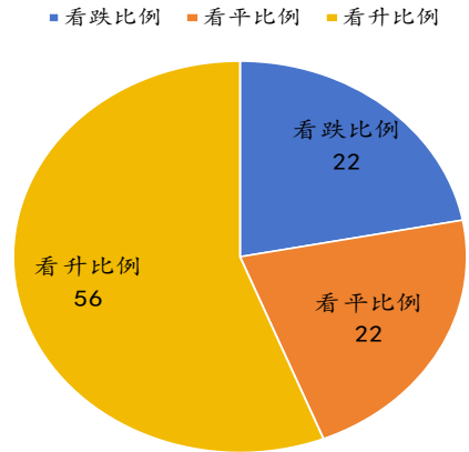
中国LNG心态调查（周度）-%
