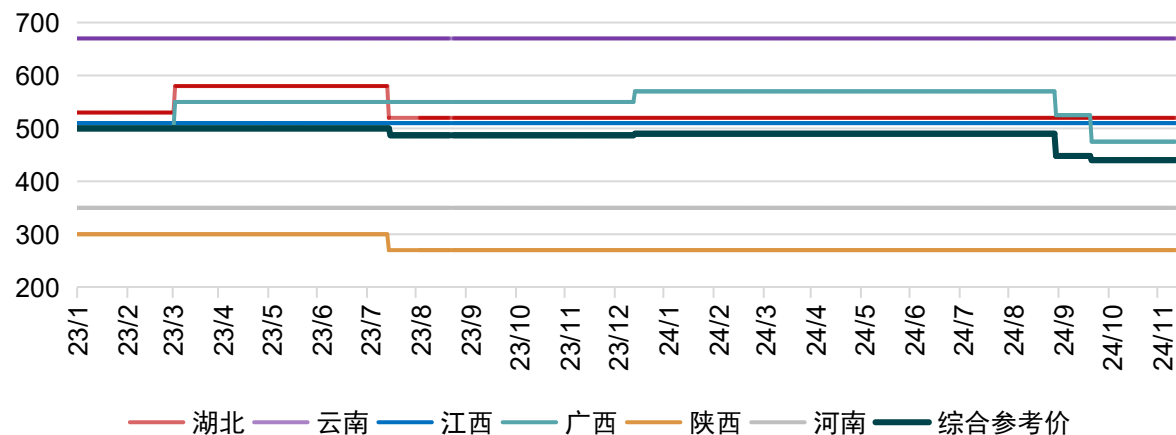
硅煤价格
