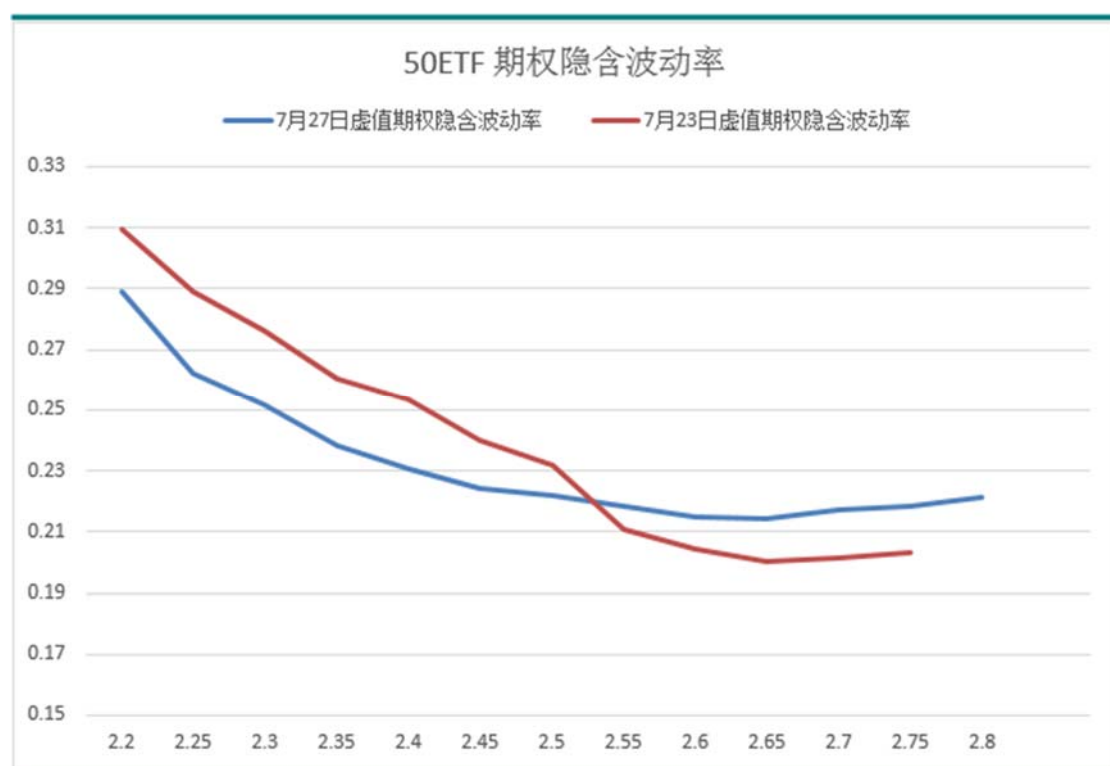
图表 7：上证 50ETF 期权隐含波动率偏度
