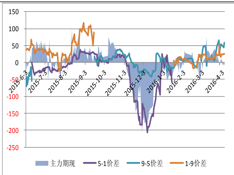
甲醇价差
